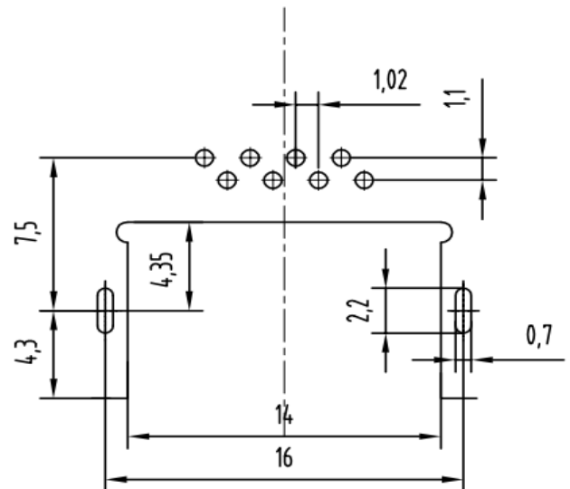
PCB参考图
