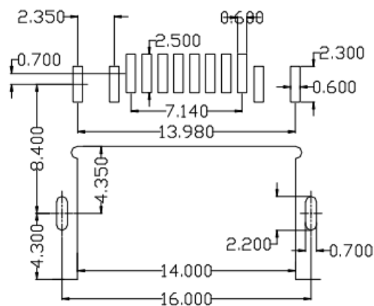
PCB参考图
